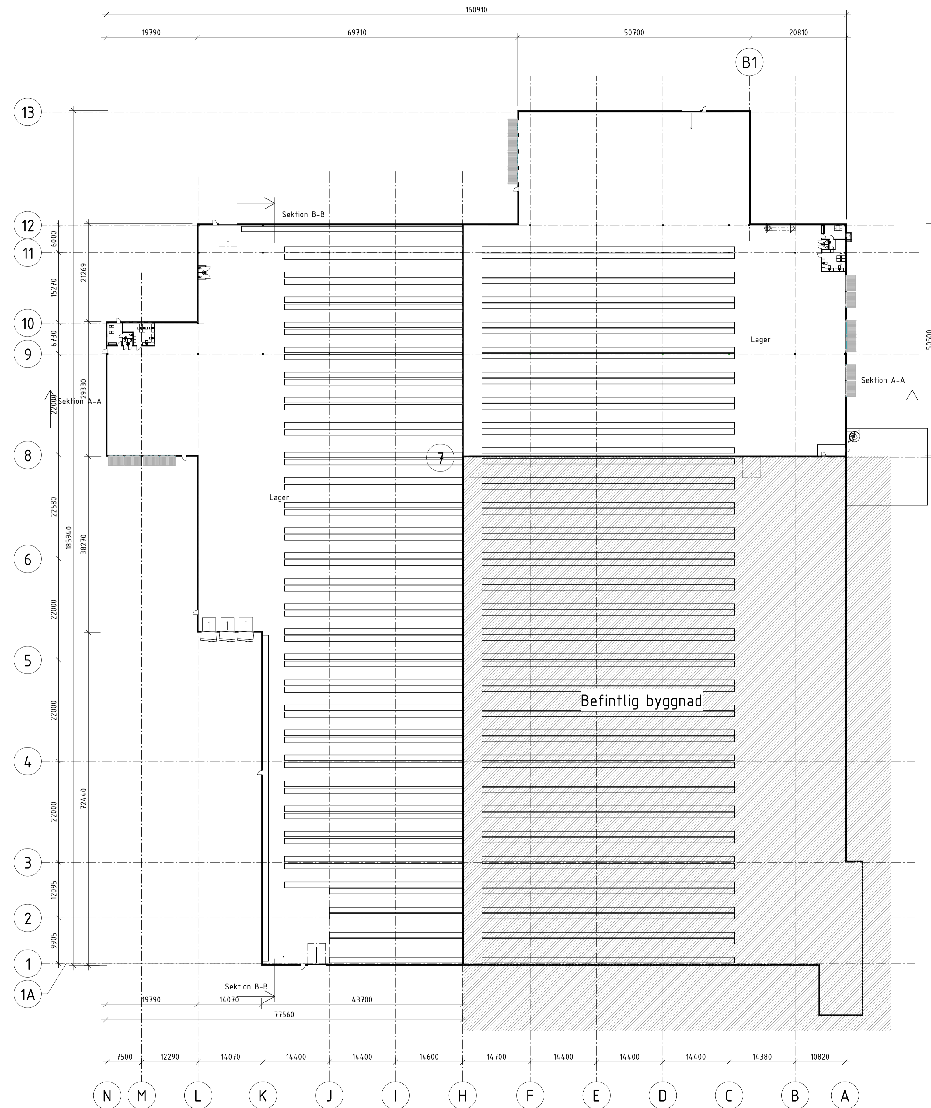
Plan 1 1 : 500
