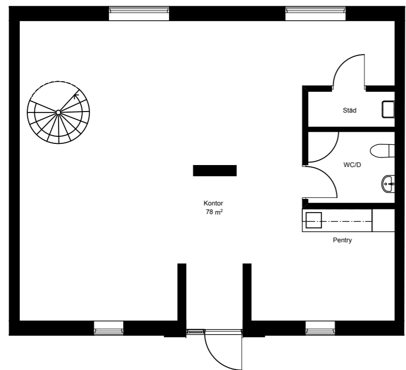
0. Våning 0 Lokal 1:100
