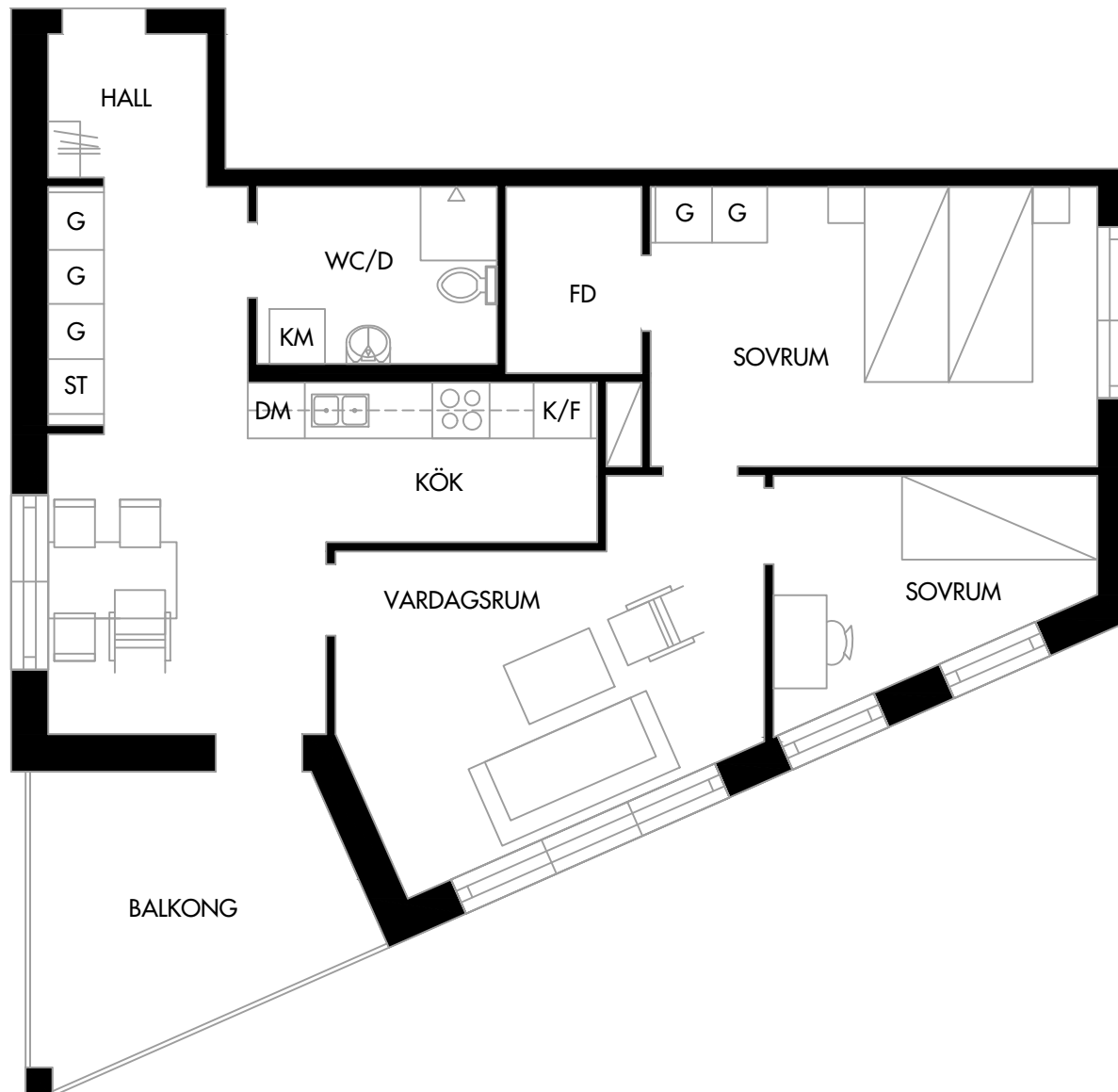
D-136 Plan 13 3 Rok , 72.5 m 2
