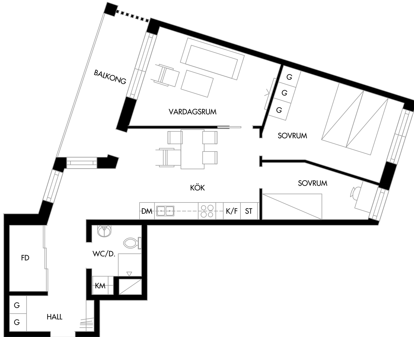
D-113 Plan 11/D-123 Plan 12 3 Rok , 71 m 2
